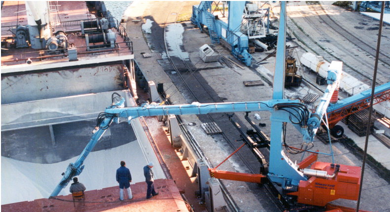
SIWERTELL ROAD-MOBILE UNLOADER - CROATIA
